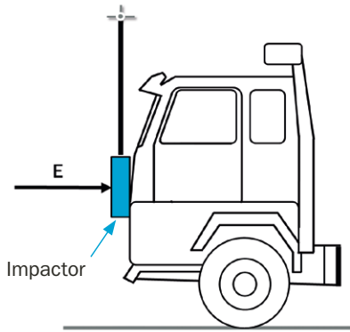
A: Front impact 1
